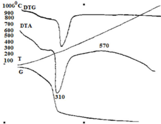
Fig. 3. DTA/TG curves of the Suulkhar iron ore.
